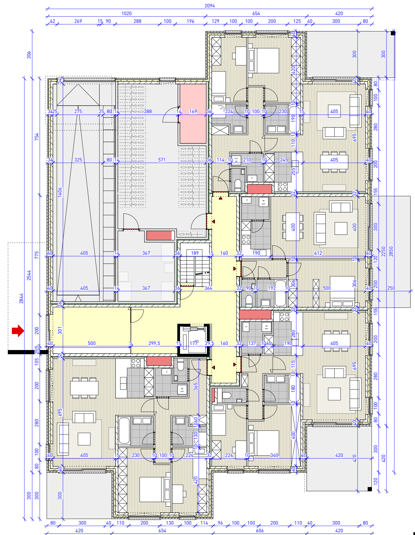
Niveau +0
