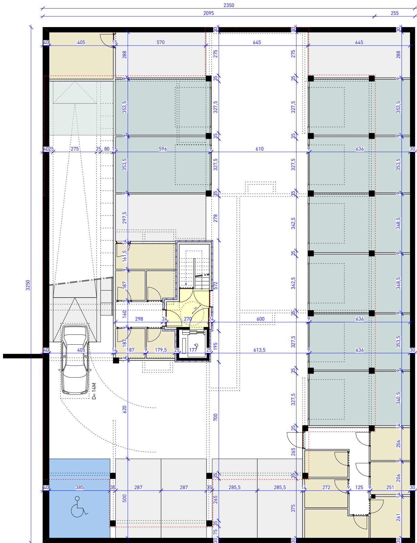
Niveau -1
